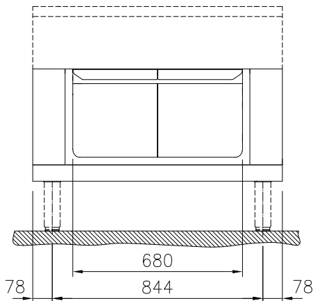
Front aanzicht
